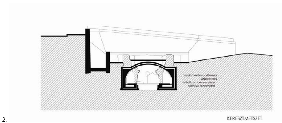
1-2. Az Ókeresztény Mauzóleum metszetei (tervezett állapot)
