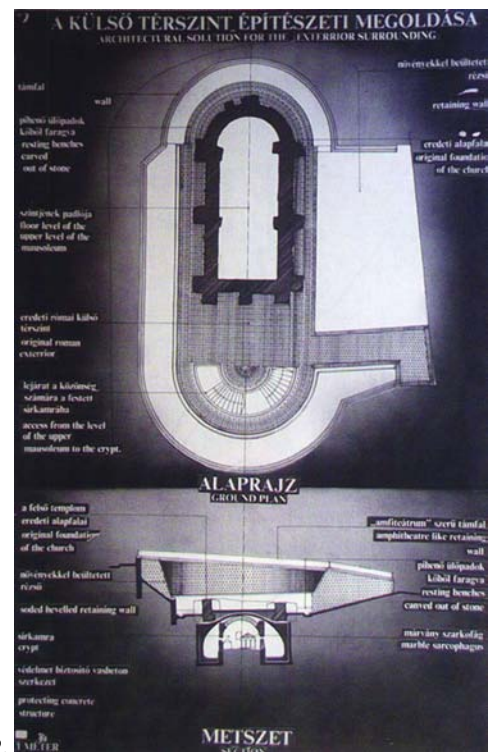
1-2. A védőépület eredeti tervei
