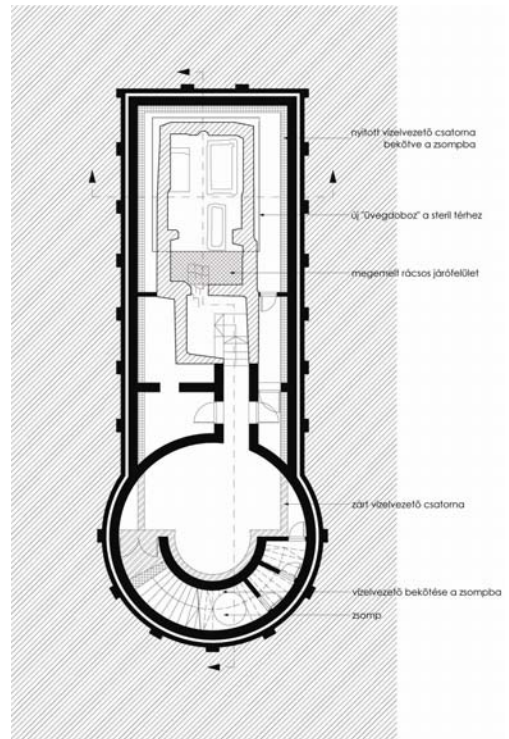
1. ALAPRAJZ
