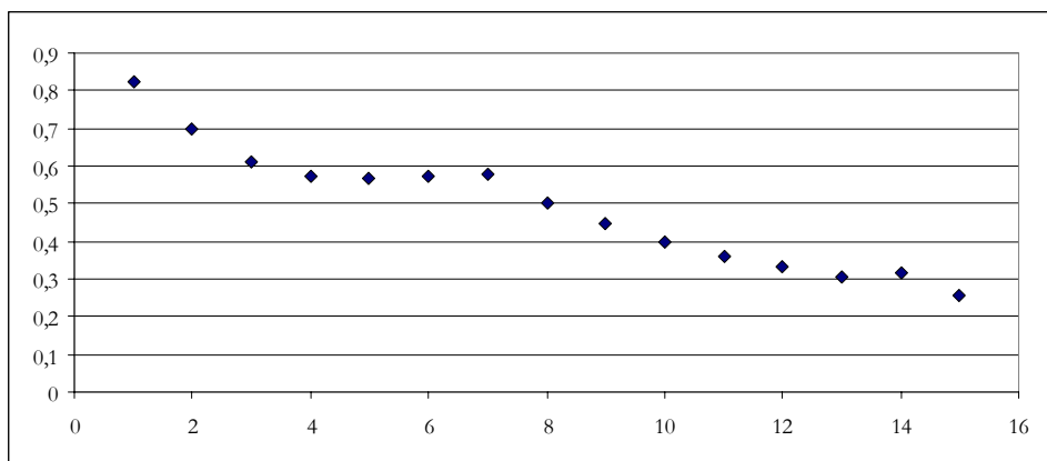
4. ábra – Az autokorrelációs függvény. Az x tengelyen az olvasható le, hogy hány nappal toltuk el az adatsort önmagához képest. Az y érték az eredeti és az eltolt adatsort korrelációja
