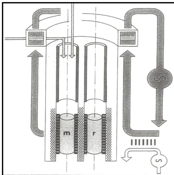
5. Ábra: A SETARAM Micro DSC-II kaloriméter celláinak sematikus elrendezése.
