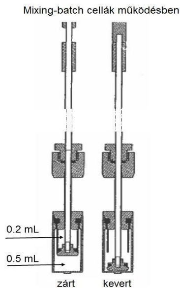
8. Ábra: Speciálisan kialakított kettős falú, sterilen zárható keverő edény.
