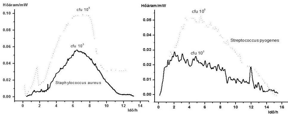
13. Ábra: A Staphylococcus aureus és a Streptococcus pyogenes szaporodása során regisztrált termikus változások 37 ° C-on.
