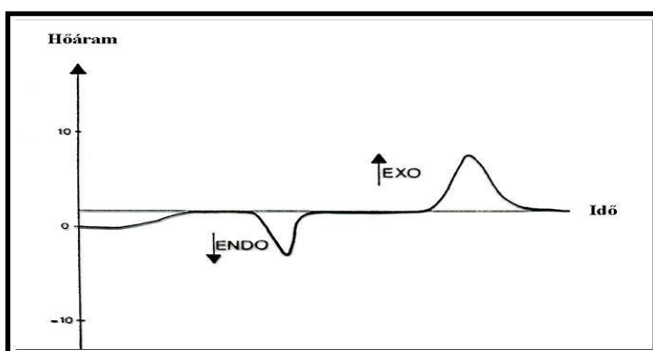
6. Ábra: A SETARAM Micro DSC-II mérhető kimenő jele.
