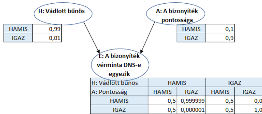
VI-3. ábra A bizonyíték a bizonyíték pontosságának figyelembevételével és a valószínűségi táblákkal 586
