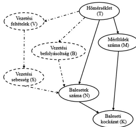
VII-7. ábra A halálos országúti balesetek Fenton és Neil szerinti kibővített oksági modellje 675
