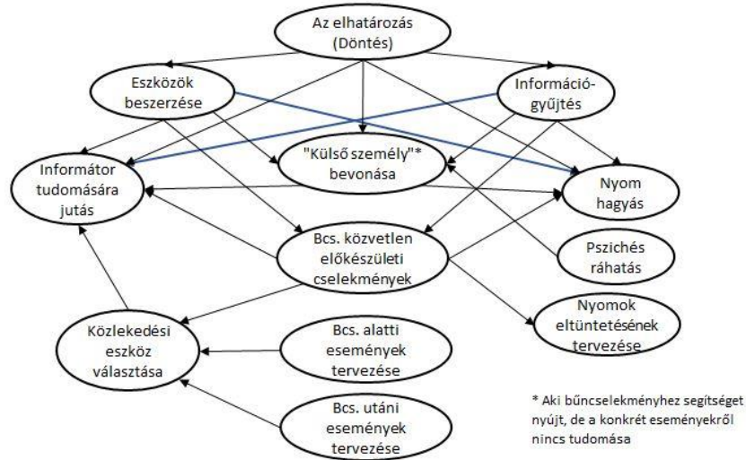
VIII-17. ábra Az elkövető viselkedésének valószínűségi hálós becslése 933
