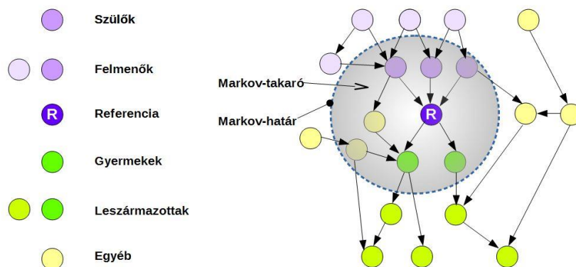
IV-8. ábra A Markov-takaró és a Markov-határ 292
