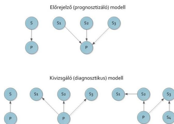
IV-7. ábra Az előrejelző (prognosztikus) és a kivizsgálási (diagnosztikus) alapmodellek ábrázolási formái (Sebastiani és Pearl alapján) 287
