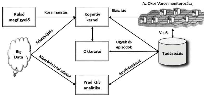
VII-16. ábra Az okos városok korai riasztási előrejelző rendszerének struktúrája 784
