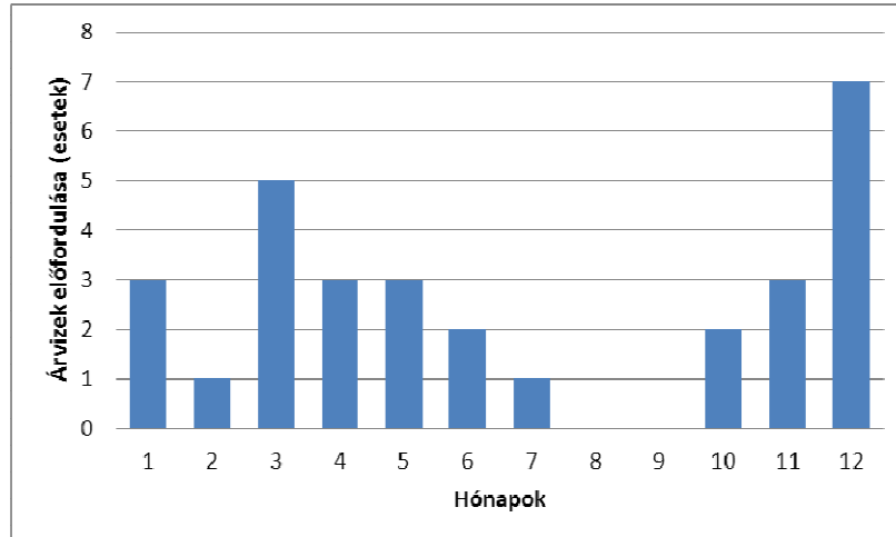
5. ábra: Árvizek előfordulása havi bontásban 1970–2009 között.
