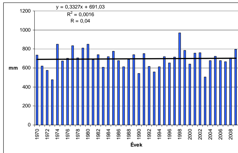
20. ábra: Az évi csapadékmennyiség változása Beregszászban 1970–2009 között.
