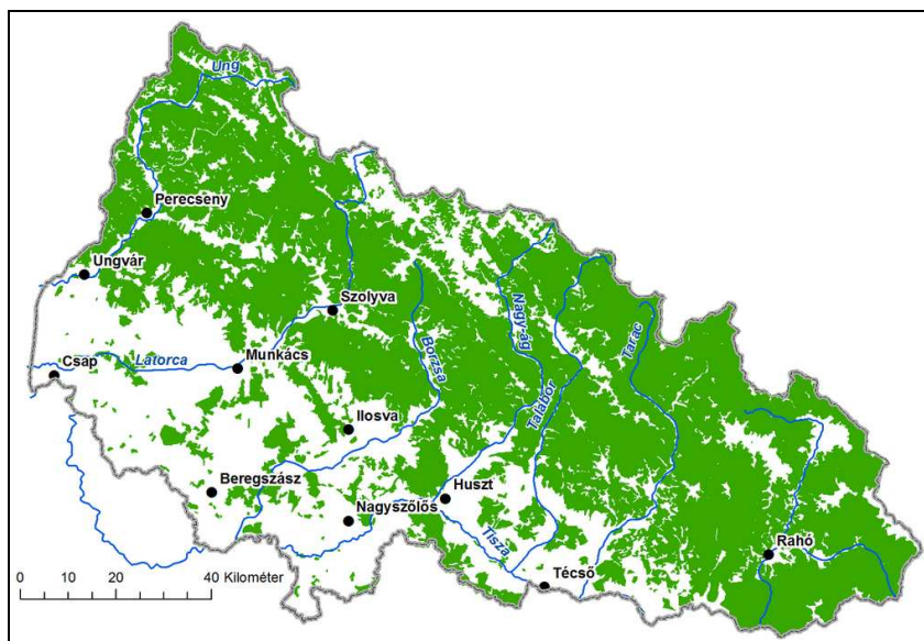
5. térkép: Kárpátalja erdővel borított területei (zöld szín – erdővel borított területek). Forrás: KÁRPÁTALJA ATLASZA 1991; Szerkesztette Molnár D.I.
