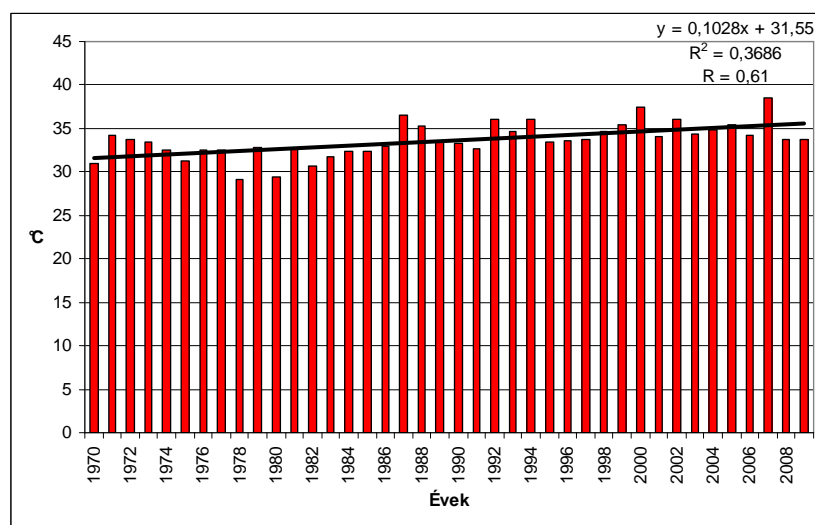
12. ábra: Az évi abszolút maximum hőmérsékletek Beregszászban 1970 és 2009 között. Forrás: BEREGSZÁSZI METEOROLÓGIAI ÁLLOMÁS adattára, 2010; Szerkesztette Izsák T.
