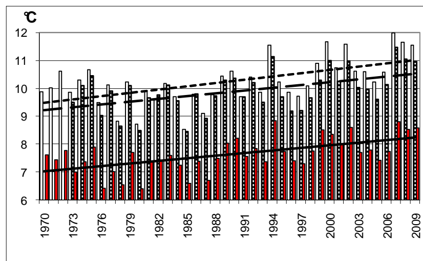
18. ábra: A beregszászi, ungvári és rahói évi középhőmérsékletek alakulása az 1970–2009-es időszakban. (Középhőmérséklet: Beregszász - üres oszlopok, Ungvár - csíkos oszlopok, Rahó - kitöltött oszlopok; trendegyenesek: Beregszász szaggatott, Ungvár hosszabbra szaggatott, Rahó folytonos vonal)
