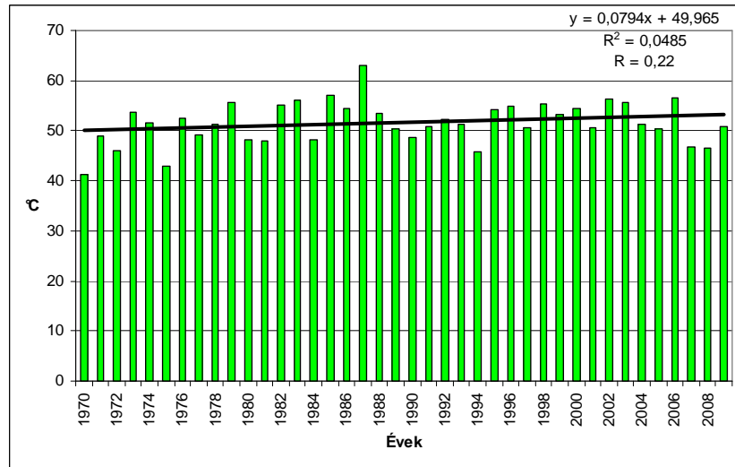
16. ábra: Évi abszolút hőingás Beregszászban 1970–2009 között.
