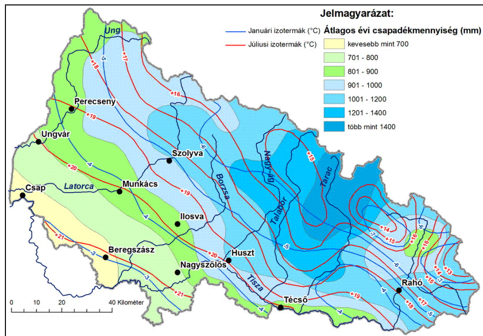
3. térkép: Kárpátalja éghajlata. Forrás: KÁRPÁTALJA ATLASZA 1991.
