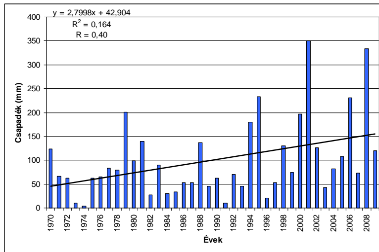
6. ábra: A csapadékmennyiség változása Rahón 1970–2009 között március hónapokban. Forrás: KÁRPÁTALJAI HIDROMETEOROLÓGIAI KÖZPONT adattára, 2010; Szerkesztette Izsák T.
