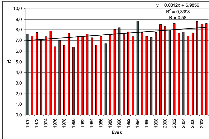
11. ábra: Sokévi átlagos középhőmérsékletek Rahón 1970–2009 között. Forrás: KÁRPÁTALJAI MEGYEI HIDROMETEOROLÓGIAI KÖZPONT adattára, 2010; Szerkesztette Izsák T.
