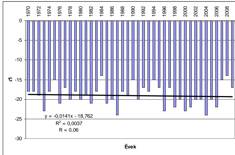
15. ábra: Az évi abszolút minimum hőmérsékletek Rahón 1970–2009 között. Forrás: KÁRPÁTALJAI MEGYEI HIDROMETEOROLÓGIAI KÖZPONT adattára, 2010; Szerkesztette Izsák T.
