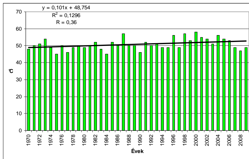
17. ábra: Évi abszolút hőingás Rahón 1970–2009 között.
