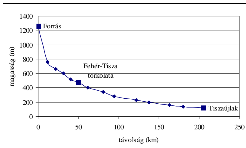
2. ábra: A Tisza esésgörbéje a Fekete-Tisza forrásától Tiszaújlakig. Forrás: NAGY B. et al. 2002.
