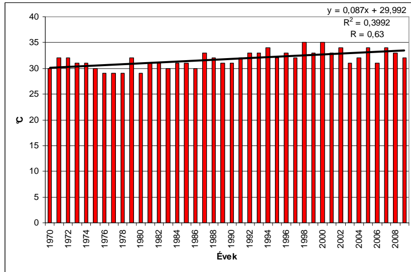
13. ábra: Az évi abszolút maximum hőmérsékletek Rahón 1970 és 2009 között. Forrás: KÁRPÁTALJAI MEGYEI HIDROMETEOROLÓGIAI KÖZPONT adataira, 2010; Szerkesztette Izsák T.
