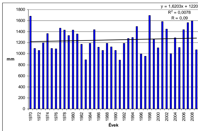
21. ábra: Az évi csapadékmennyiség változása Rahón 1970–2009 között. Forrás: KÁRPÁTALJAI MEGYEI HIDROMETEOROLÓGIAI KÖZPONT adattára, 2010; Szerkesztette Izsák T.
