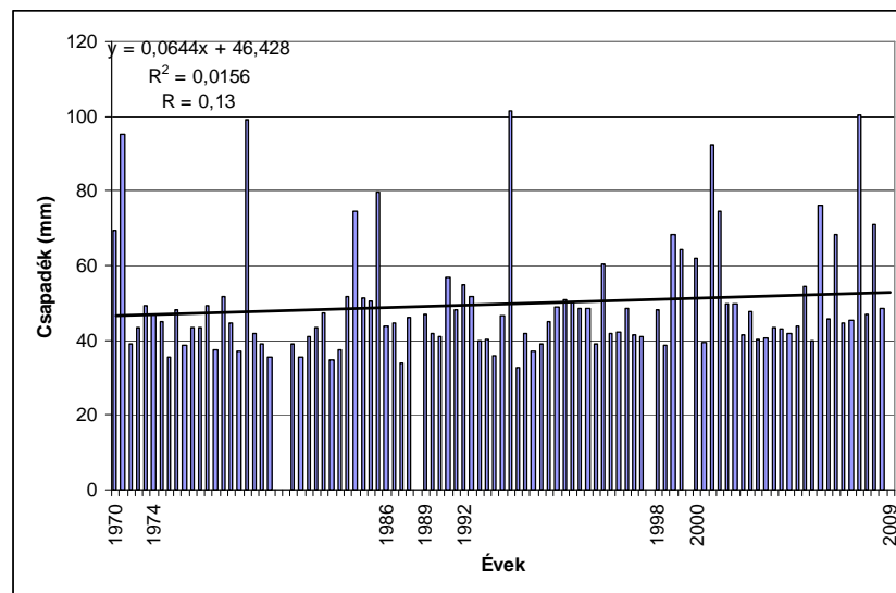
22. ábra: A csapadék 40 mm/nap fölötti értékeinek változása Rahón 1970–2009 között. Forrás: KÁRPÁTALJAI MEGYEI HIDROMETEOROLÓGIAI KÖZPONT adattára, 2011; Szerkesztette Izsák T.
