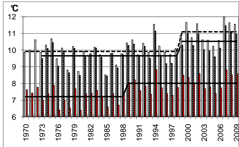
19. ábra: A beregszászi, ungvári és rahói évi középhőmérsékletek alakulása az 1970–2009-es időszakban. (Középhőmérséklet: Beregszász - üres oszlopok, Ungvár - csíkos oszlopok, Rahó - kitöltött oszlopok; a megtört vízszintes szakaszok az idősorokban detektált szignifikáns töréspontok által elválasztott részátlagokat jelenítik meg: Beregszász - rövidre szaggatott, Ungvár - hosszabbra szaggatott, Rahó - folytonos vonal)
