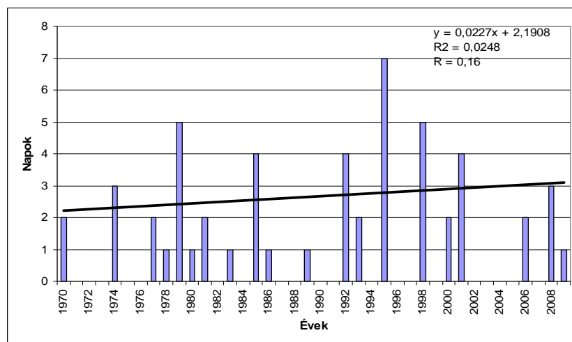
8. ábra: A hullámtér vízzel való borítottsága (napok száma) Tiszaújlaknál az árvizek idején 1970–2009 között.
