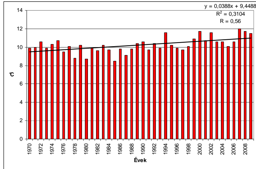
10. ábra: Sokévi átlagos középhőmérsékletek Beregszászban 1970–2009 között. Forrás: BEREGSZÁSZI METEOROLÓGIAI ÁLLOMÁS adattára, 2010; Szerkesztette Izsák T.
