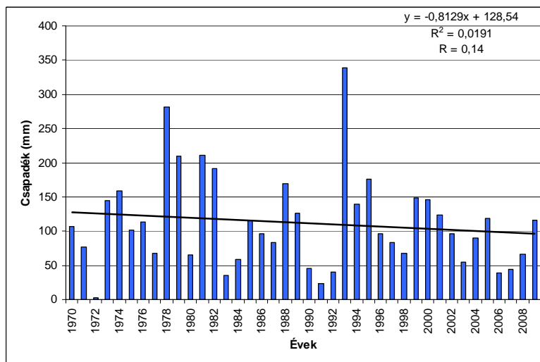
7. ábra: A csapadékmennyiség változása Rahón 1970–2009 között december hónapokban. Forrás: KÁRPÁTALJAI HIDROMETEOROLÓGIAI KÖZPONT adattára, 2010; Szerkesztette Izsák T.
