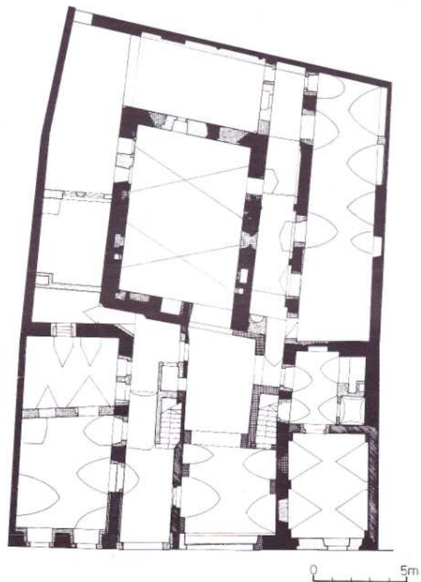
28. ábra. Az Újutca 22-24. sz. telek földszinti beépítése 1972-ben, a falak kormeghatározásával
