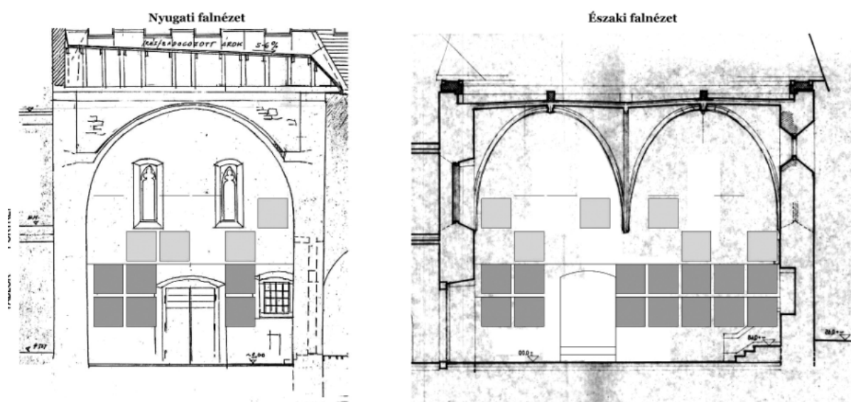
59-60. ábra. A volt magánzsinagóga terének nyugati és északi falnézetei
